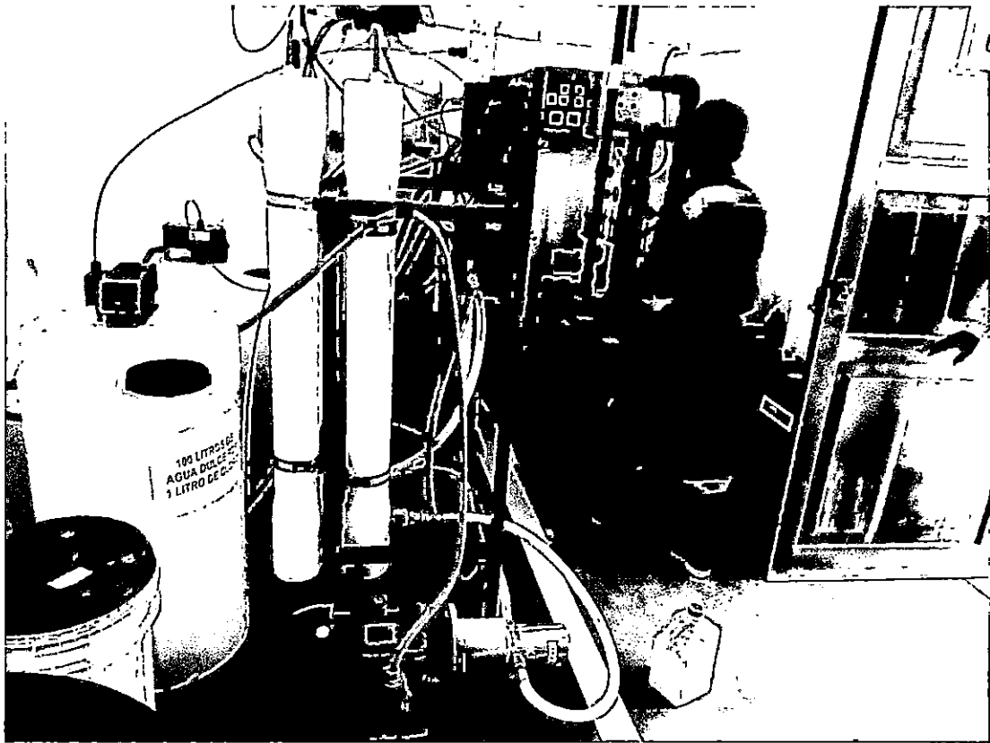
Fotografía N°21: Vista de estado de planta de ósmosis inversa.
